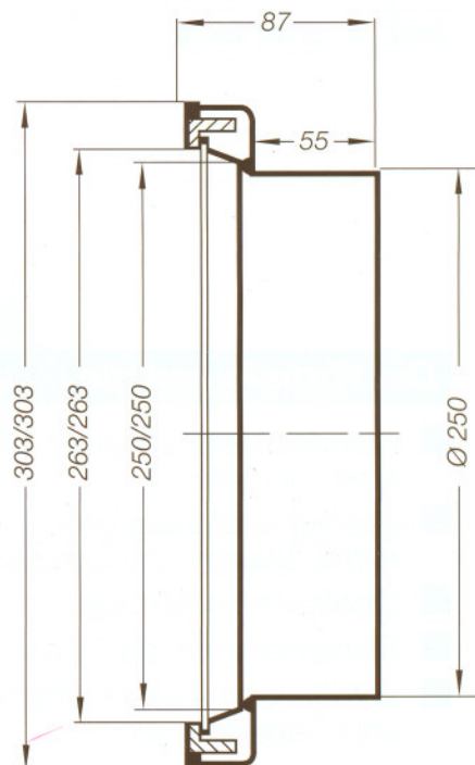
Einbaudose Typ 358
